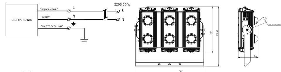
Рисунок 1. Электрическая схема подключения.
